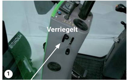
Transportsicherung in verriegelter Stellung.
