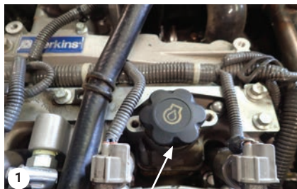
Påfyldningsdæksel, motorolie
