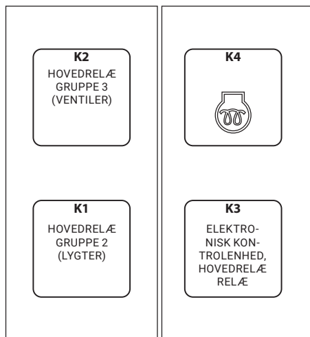
Sikringer og relæer
