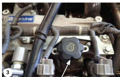
Påfyldningsdæksel, motorolie
