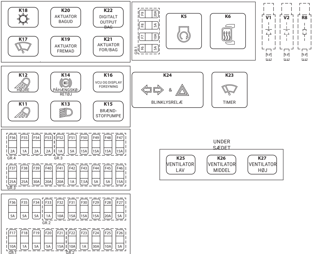
Kabinens stikdåse
