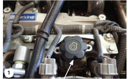
Tapón de reposición de aceite del motor
