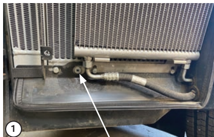
Bouchon de vidange
