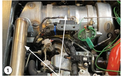
Tuyau d'échappement et DOC/DPF (Diesel Oxidation Catalyst/Diesel Particle Filter ou catalyseur d'oxydation diesel/filtre à particules diesel)
